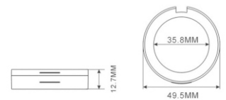
HG7224A SIZE: W49.5*H12.7MM
