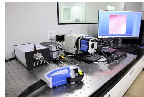
拉曼光谱仪
