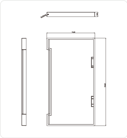
下盖
