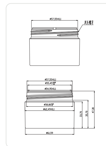
罐底
