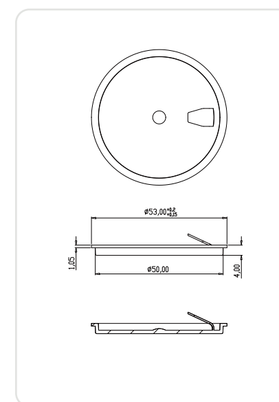
防溢盖
