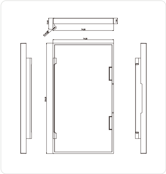
上盖
